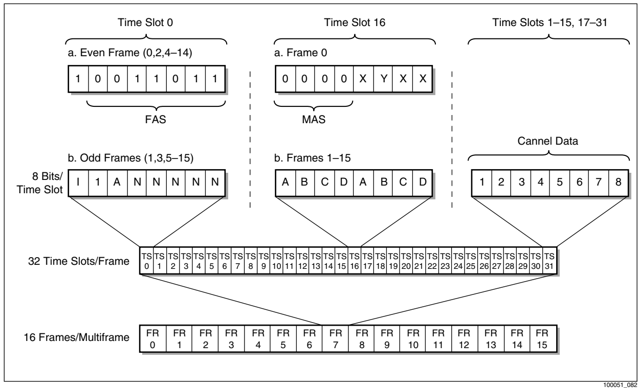
Figure A-3. E1 Format
