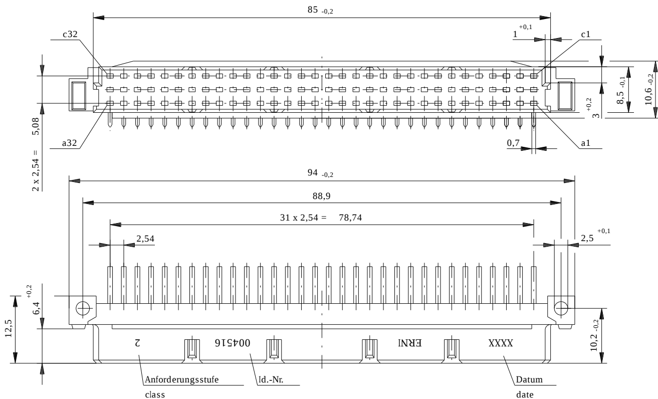
Bestückungsplan / contact layout
