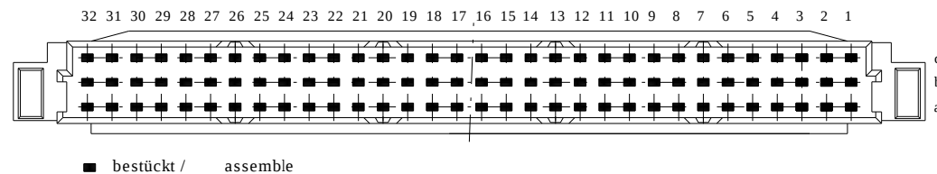
Bestückungsplan / contact layout
