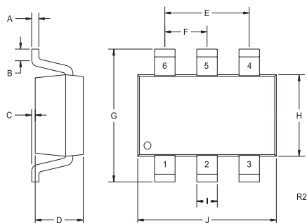
SOT-26
