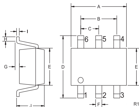
SOT-363
