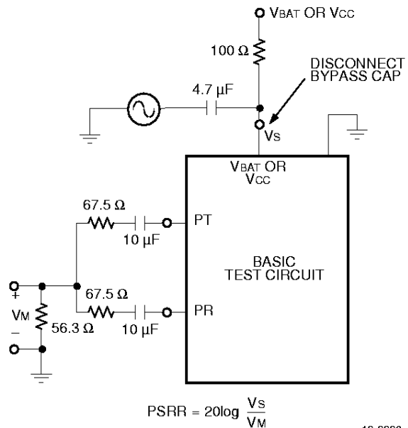
Figure 7. Longitudinal PSRR
