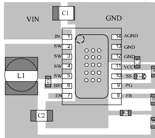
Top Layer
